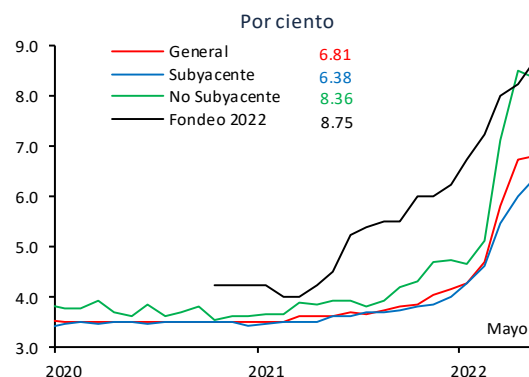
Gráfica 97 Medianas de las Expectativas de Inflación General, Subyacente, No Subyacente y Tasa de Fondo Bancario al Cierre de 2022
